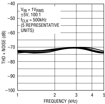
LTC1164-5 • G21
