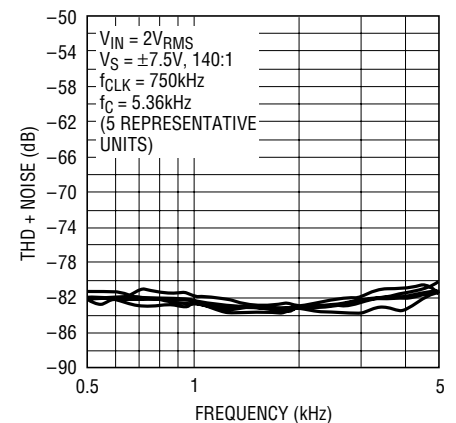
LTC1164-5 • G23
