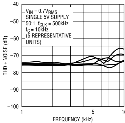
LTC1164-5 • G22
